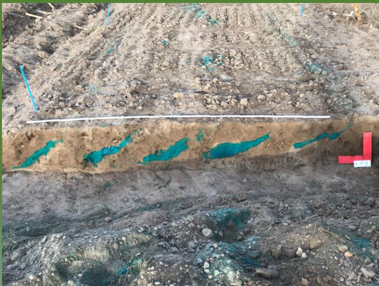
Vertikale Bodenquerschnitte
